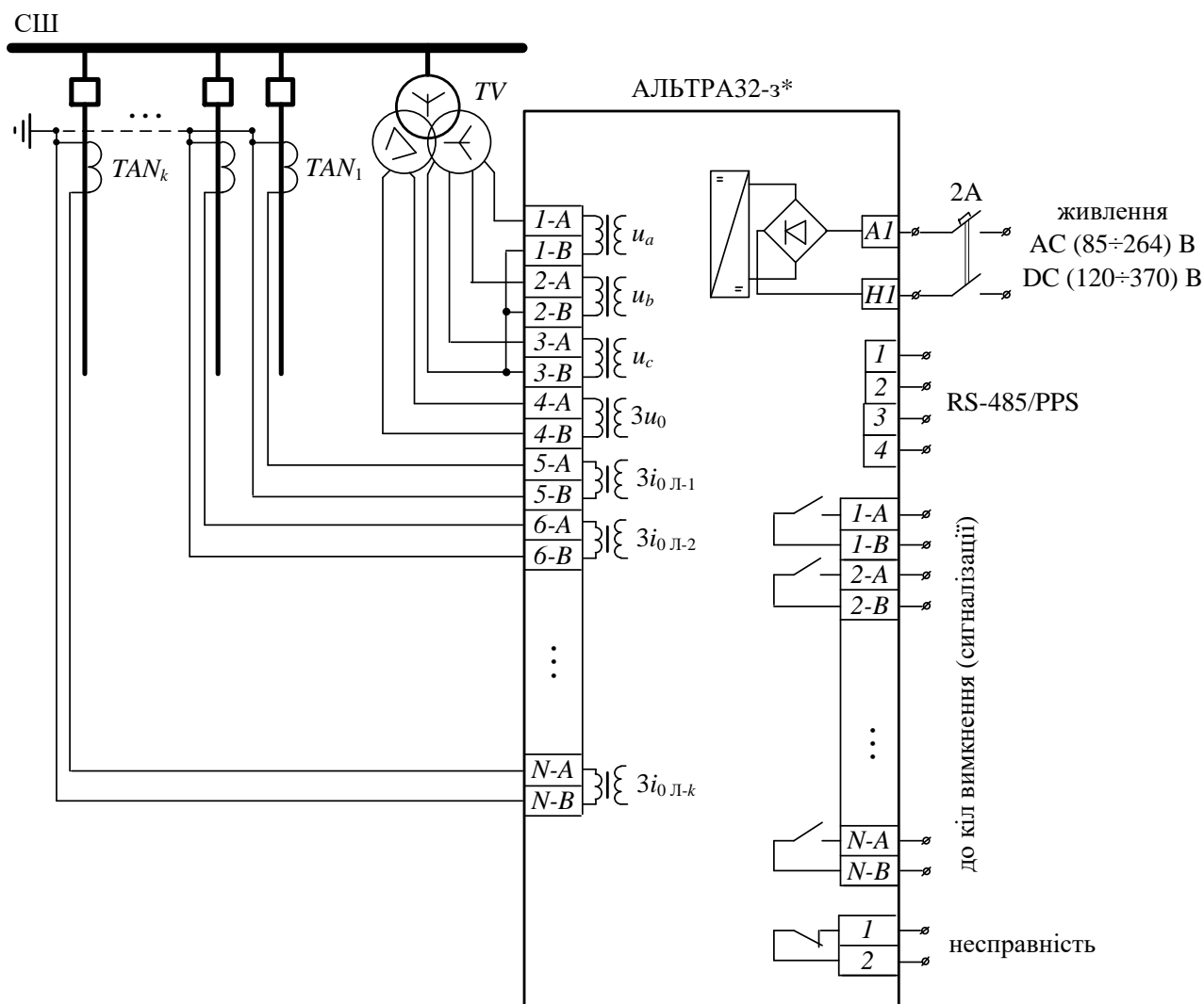
Рис. 16. Схема під'єднання пристрою АЛЬТРА32-3* до зовнішніх кіл ( N=16 або 32 )
