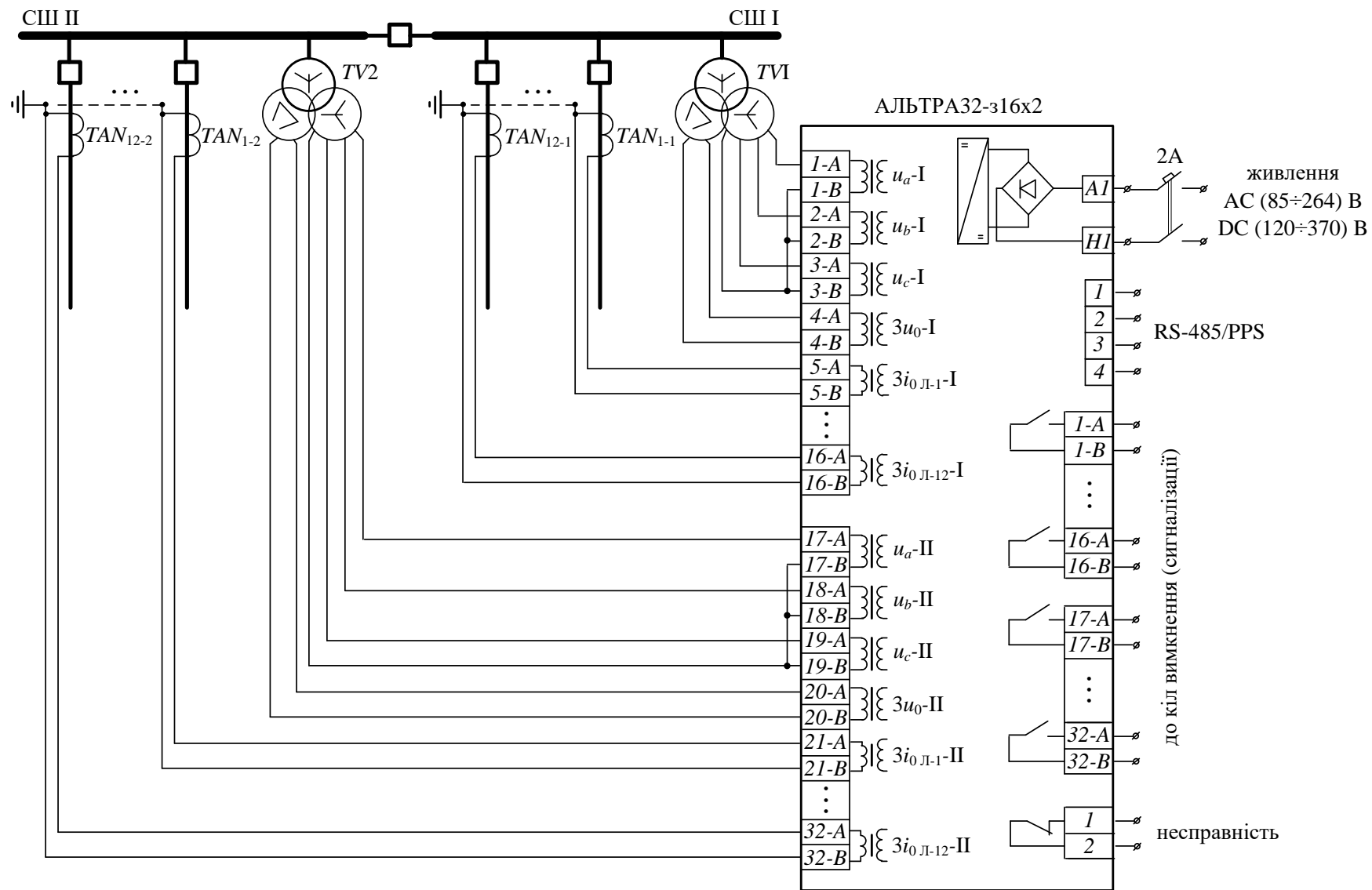
Рис. 17. Схема під'єднання пристрою АЛЬТРА32-316x2 до зовнішніх кіл
