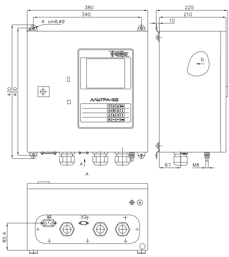
Рис. 2. Габаритні розміри пристрою АЛТРА32-332
