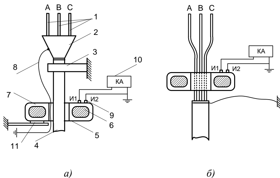
Рис. 19. Схема виконання розробки кінця кабелю та воронки
