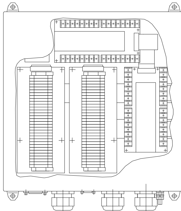
Рис. 6. Монтажна панель пристрою АЛЬТРА32-332
