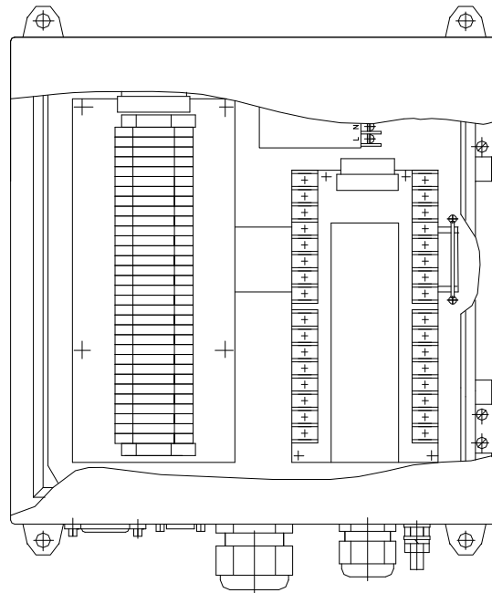
Рис. 5. Монтажна панель пристрою АЛЬТРА32-316
