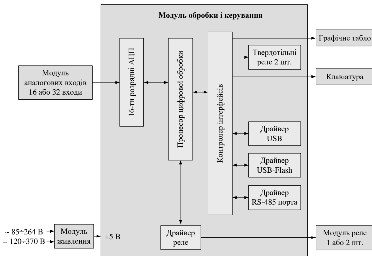
Рис. 7. Функціональна схема пристрою Альтра32-3*
