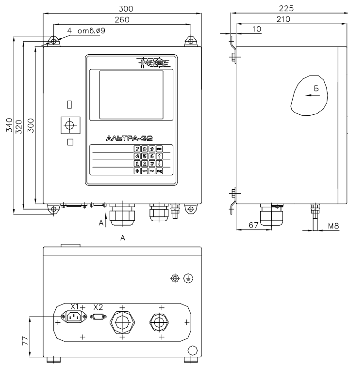
Рис. 1. Габаритні розміри пристрою АЛТРА32-з16
