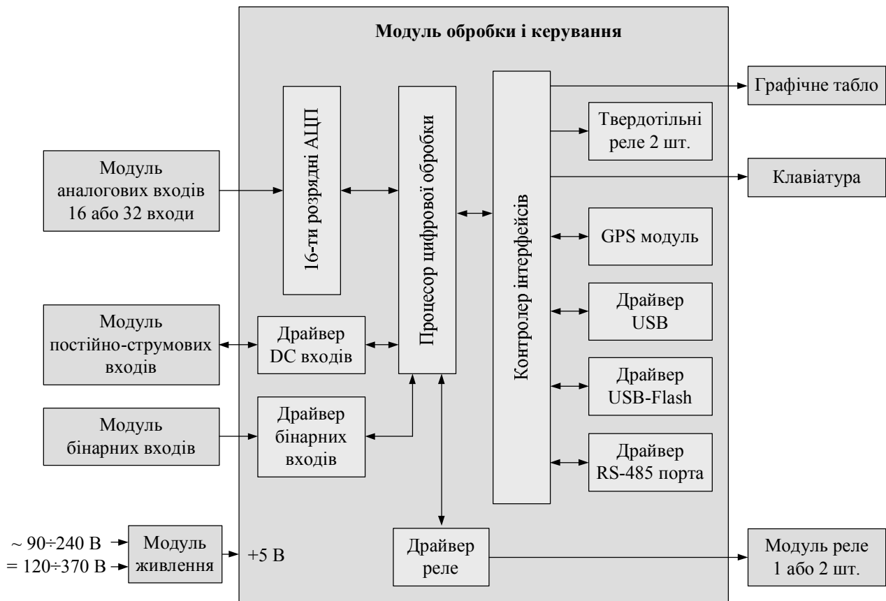
Рис. 5. Функціональна схема пристрою Альтра32
