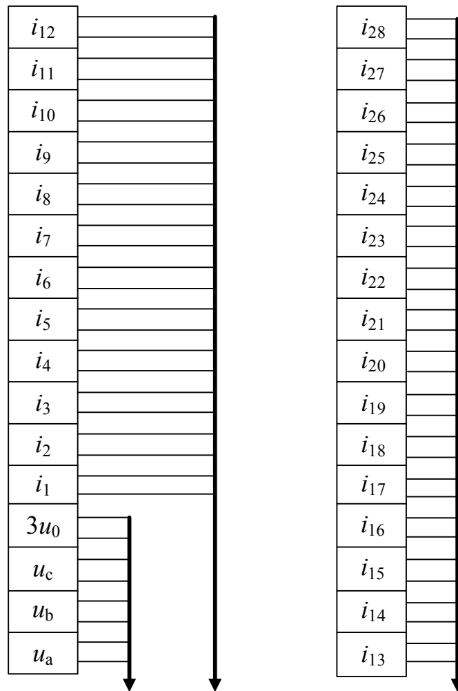
Рис. 15. Під'єднання зовнішніх аналогових кіл до клемника Пристрою
