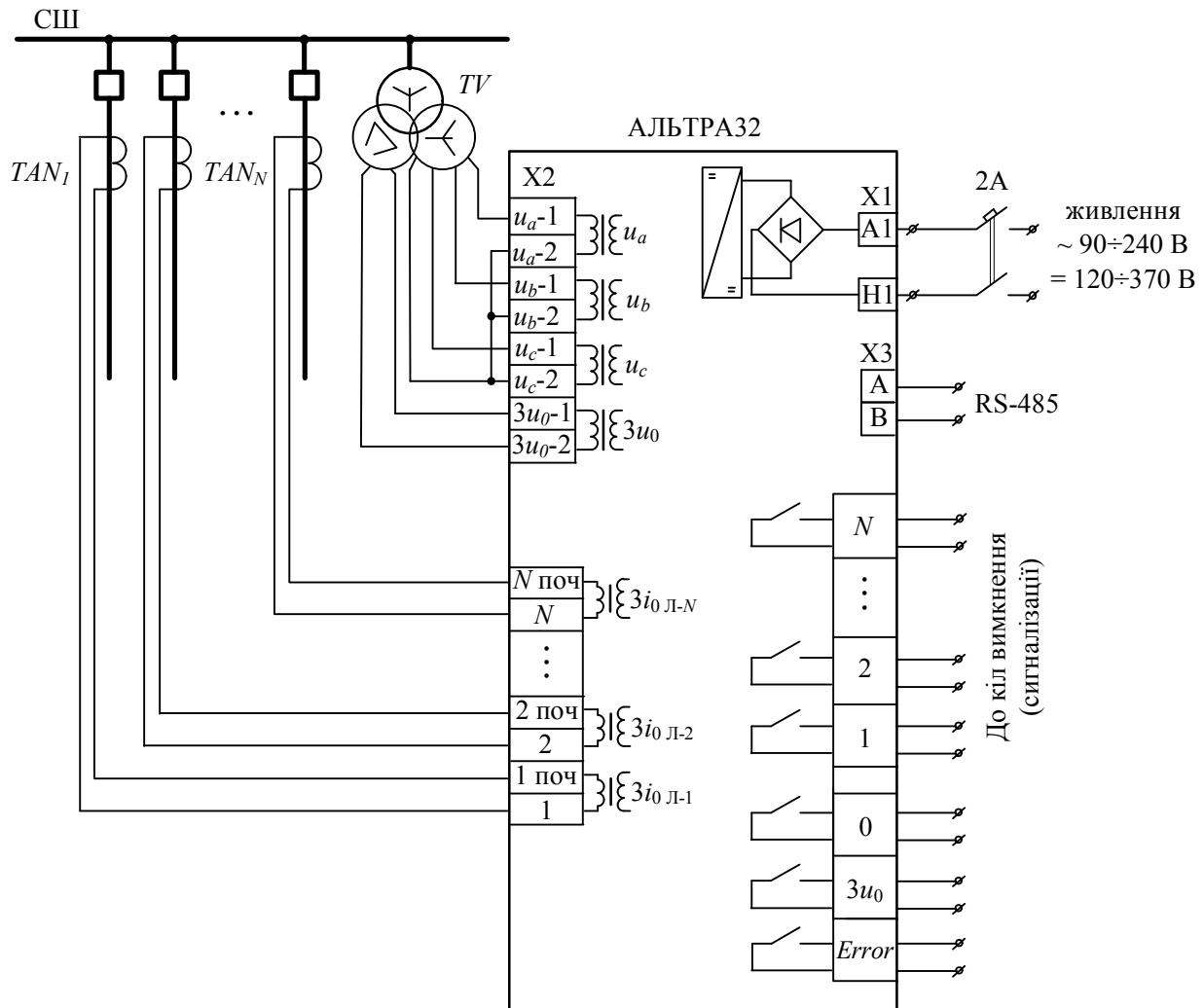
Рис. 13. Схема під'єднання пристрою АЛЬТРА32-з** до зовнішніх кіл ( N=16 або 32 ) (примітка: початок – це вивід струмових кіл, маркований кольоровою трубкою)
