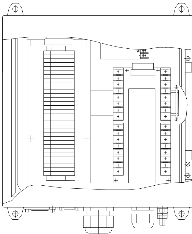
Рис. 3. Монтажна панель пристрою АЛТРА32-з16
