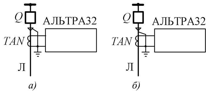
Рис. 16. Схеми під'єднання Пристрою до трансформаторів струму нульової послідовності: а – до воронки; б – до кінця розробки кабелю
