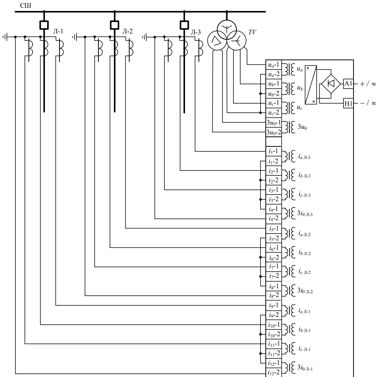
Рис. 14. Схема під'єднання пристрою АЛЬТРА32-р16 до зовнішніх кіл
