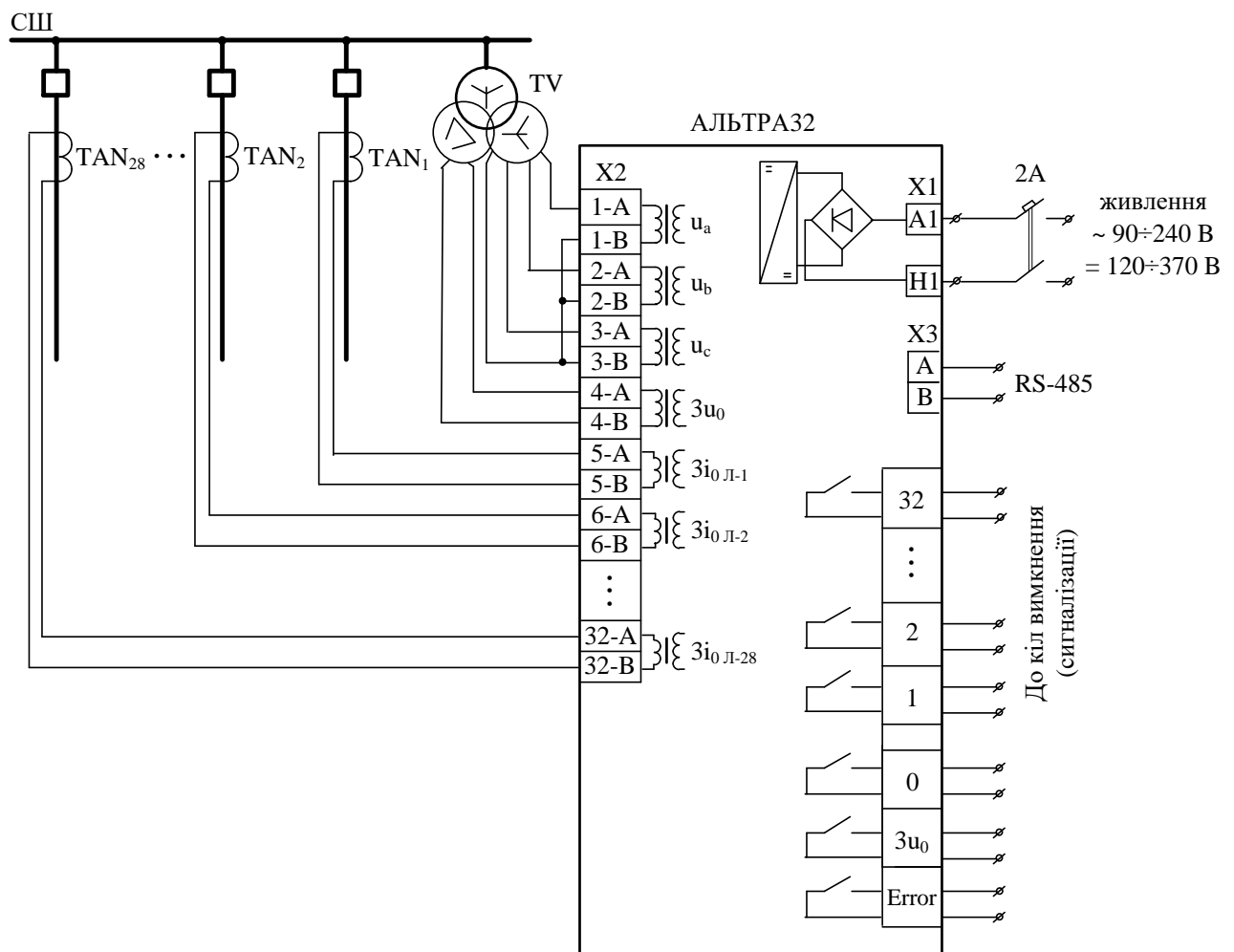
Рис. 3.5. Схема під'єднання аналогових входів Альтра32-332
