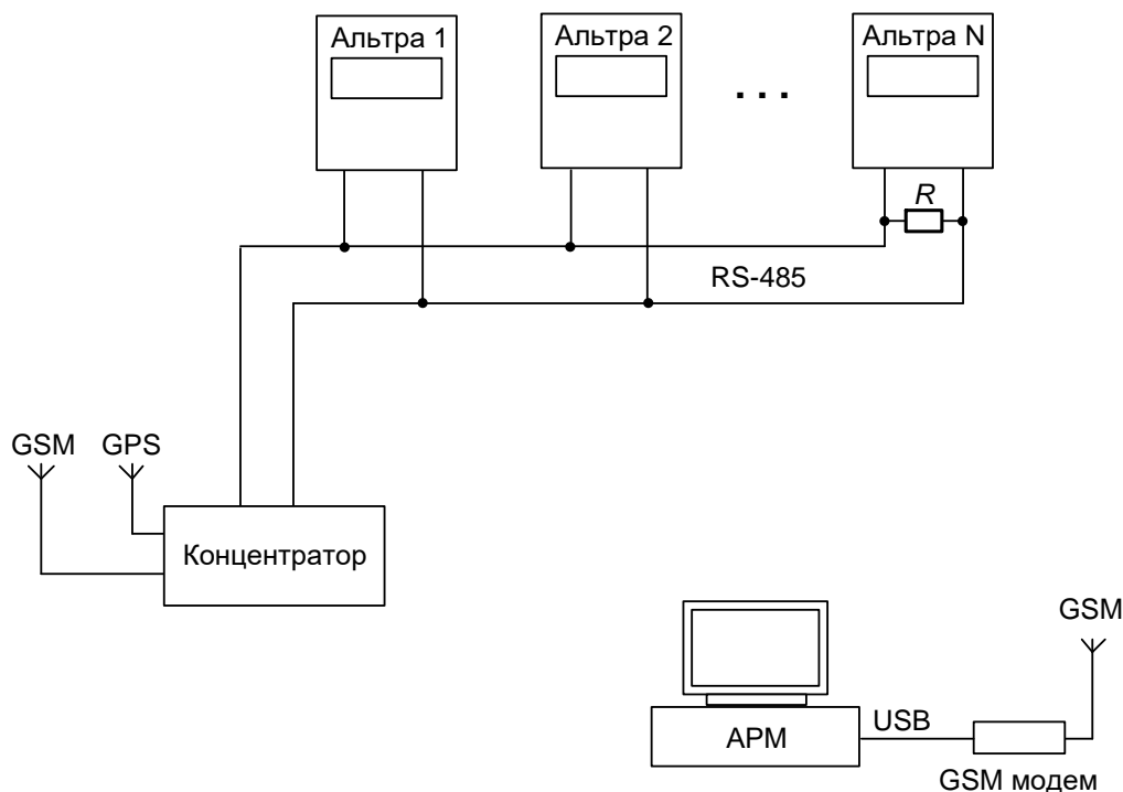
Рис. 3.27. Схема організації зв'язку з використанням GSM мережі
