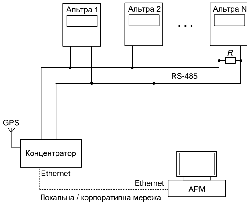
Рис. 3.22. Схема організація зв'язку з використанням Ethernet інтерфейсу
