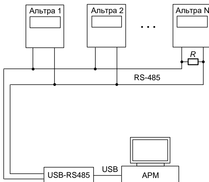
Рис. 3.21. Схема організації зв'язку з використанням RS485 інтерфейсу
