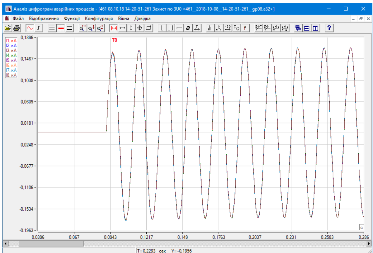
Рис. 3.17. Вигляд осцилограми струму після калібрування
