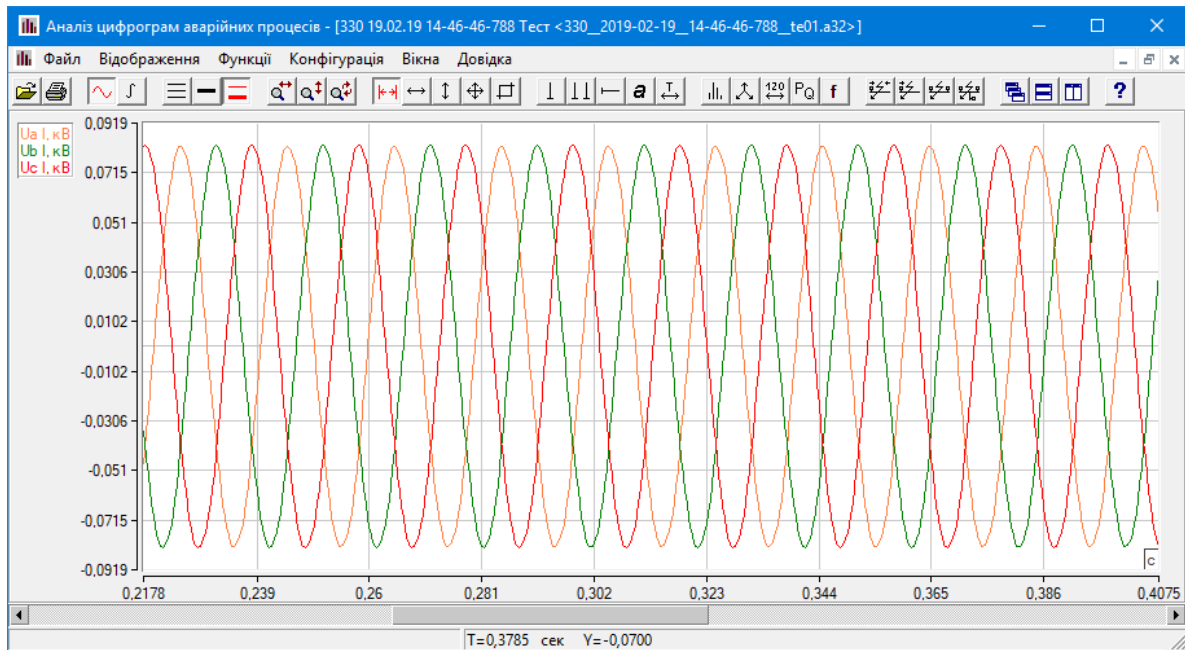
Рис. 3.19. Осцилограма з вірно фазованими каналами U_a , U_b , U_c
